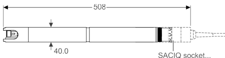
SensoLyt® 700 IQ
